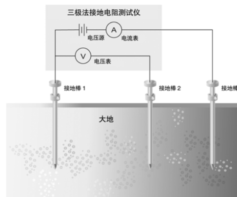
图4 三极法测试仪工作时从接地棒3到接地棒1的通路提供一个已知的电流。在电位降法电阻测试中，在通路上的不同点测量返回至被测电极接地棒2的电压。
