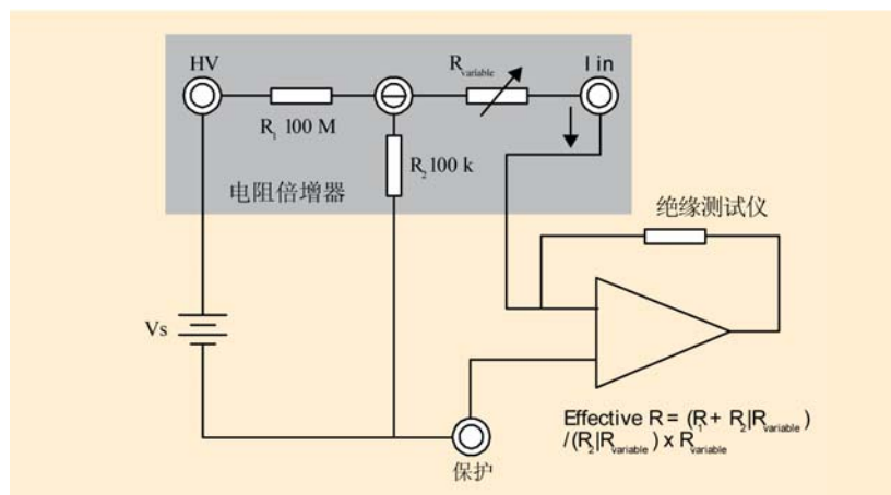
图3 将可调电阻设置为100 MΩ时，兆欧表读取的有效电阻将增大为1000倍，或者说100GΩ。
