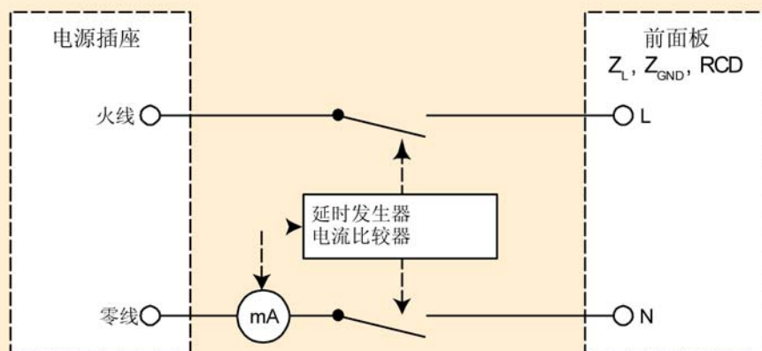
图11. 校准器的RCD功能简图 [5] 。
