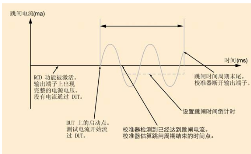
图 12. RCD 校准器的时序，它作为一个高准确度的可调 RCD。
