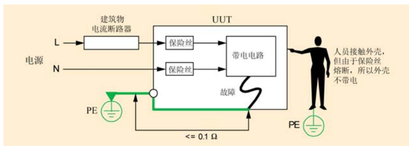
图 7. 电器的电流故障保护。
