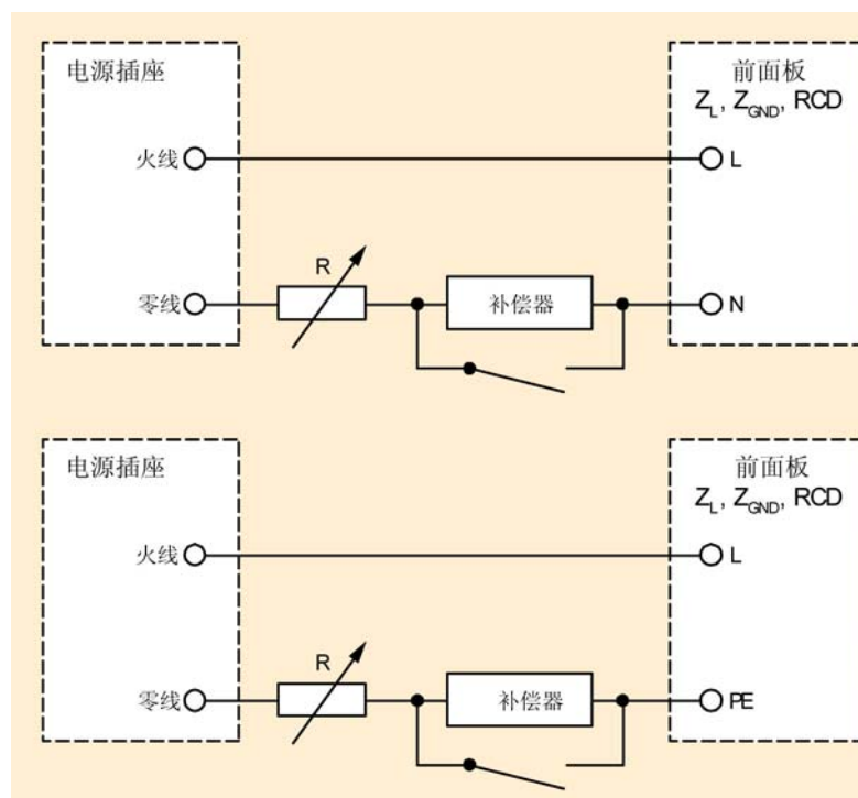
图 8. Fluke 5320A 多功能电气安全校准器的环路和线路电路简图。
